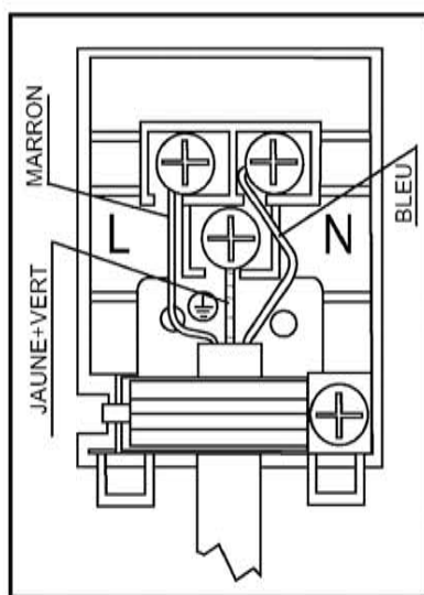
Diagramme de branchement électrique
